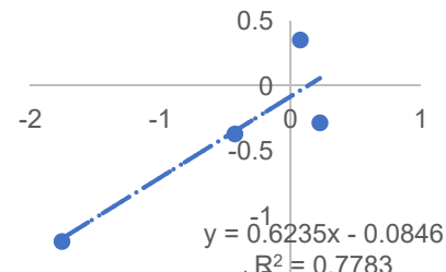
i1_LQ_BZL_c55922/f1p0/1480
